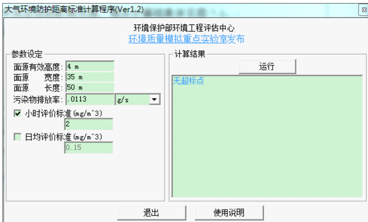
图 7-1 项目大气环境保护距离计算截图
