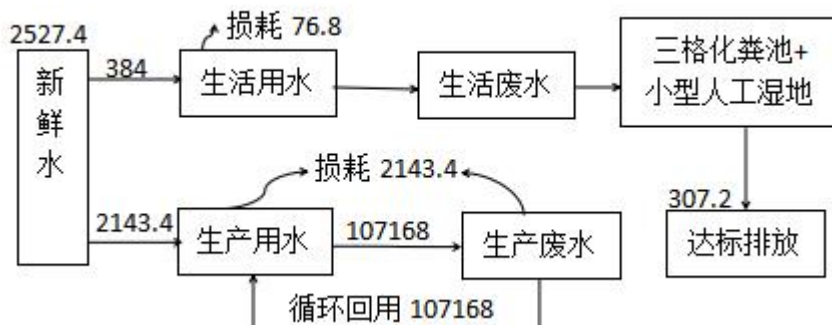
图 5-3 本项目水平衡图
