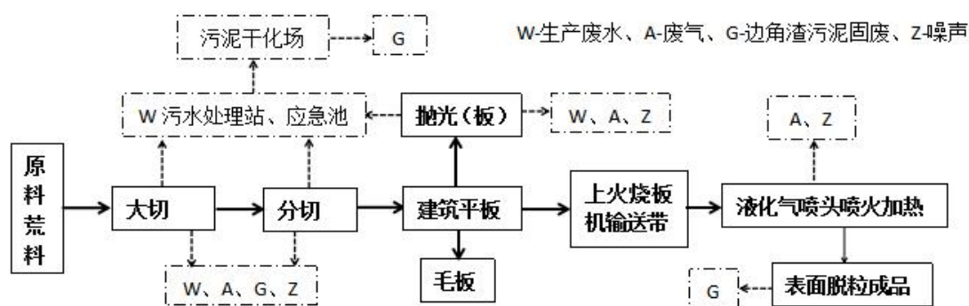
图 5-2 毛板、抛光板及火烧板工艺流程及产排污节点图
