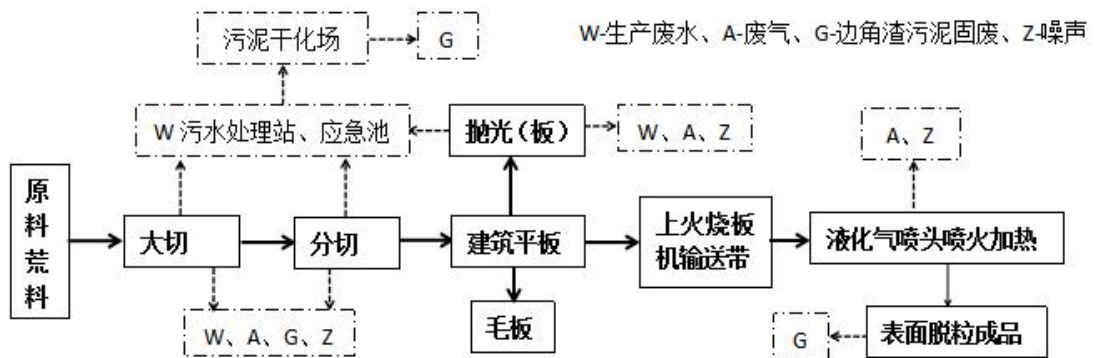
图 5-2 火烧板工艺流程及产排污节点图
