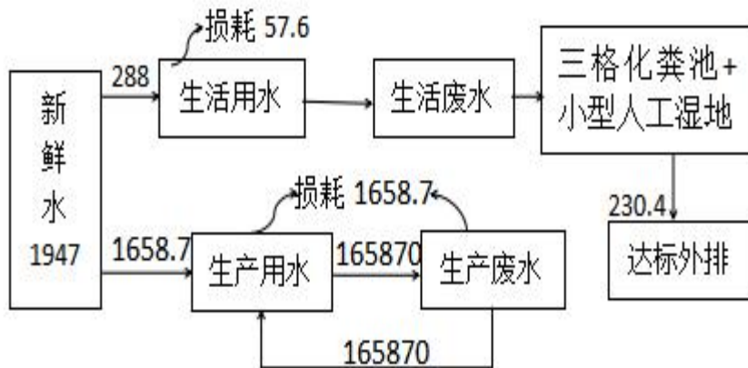
图 5-4 本项目水平衡图（单位 m 3 /a）
