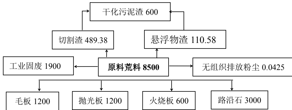
图 5-3 花岗岩物料平衡图（单位：m 3 /a）（花岗岩密度按 3t/m 3 计算）
