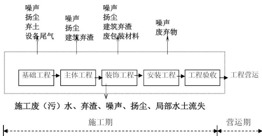
图 5-1 施工流程及产污工序图
