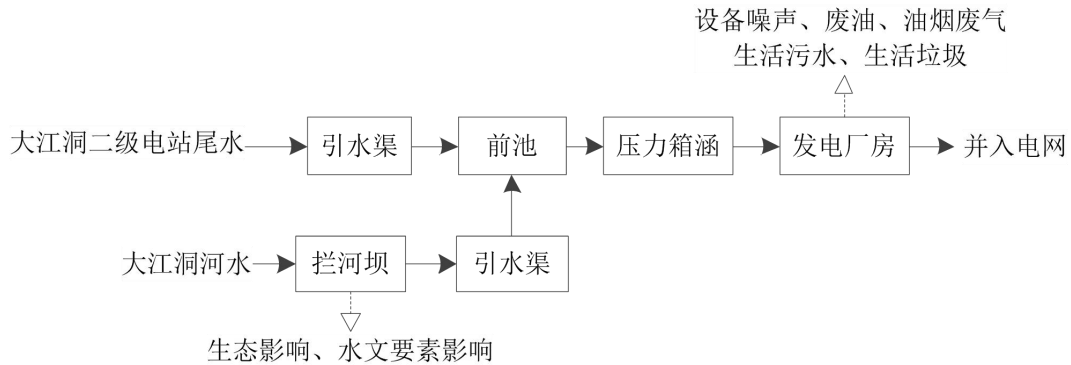
图 5-1 工艺流程及产污节点图
