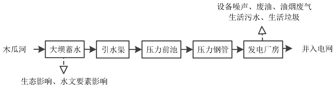
图 5-1 工艺流程及产污节点图
