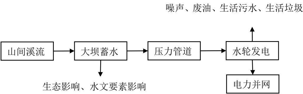
图 5-1 工艺流程及产污节点图
