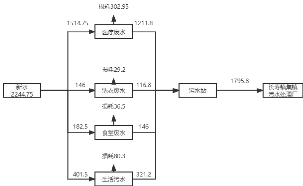
图 2-1 水平衡图 单位 m³/a
