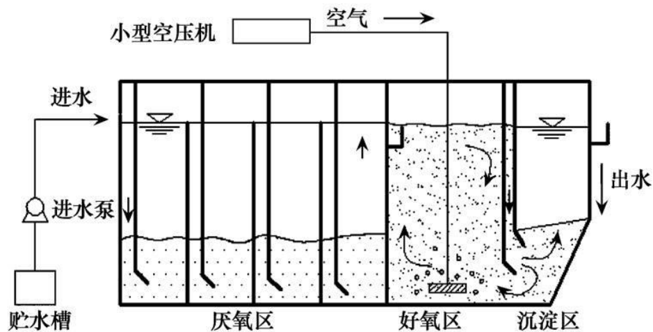
图 2-2 一体化污水处理设施示意图
