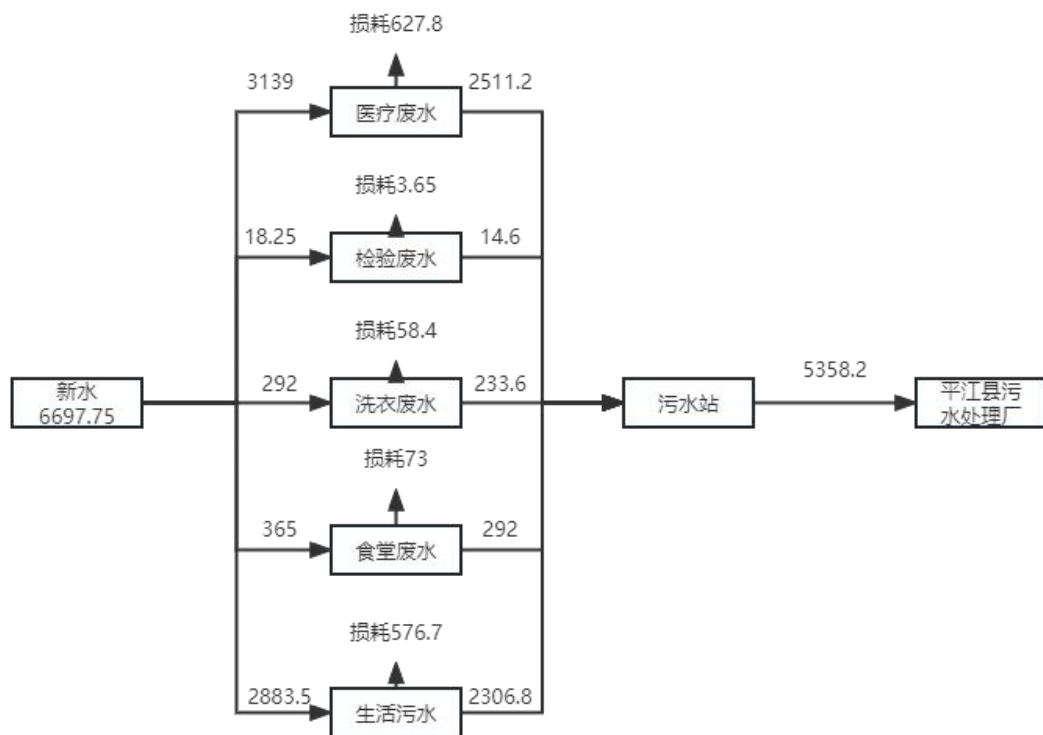
图 2-1 水平衡图 单位 \text{m}^3/\text{a}
