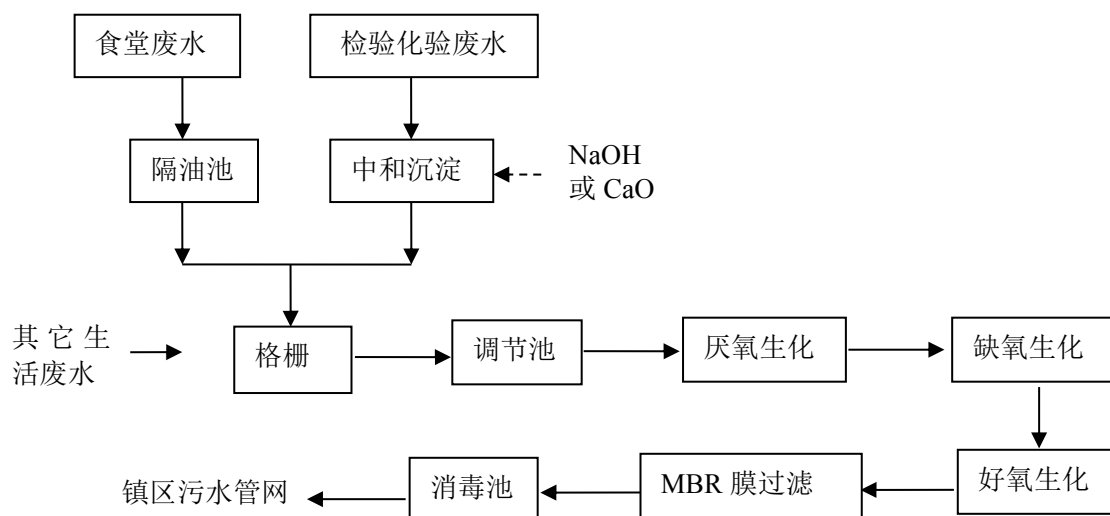
图 4-1 医院废水处理站工艺流程图
