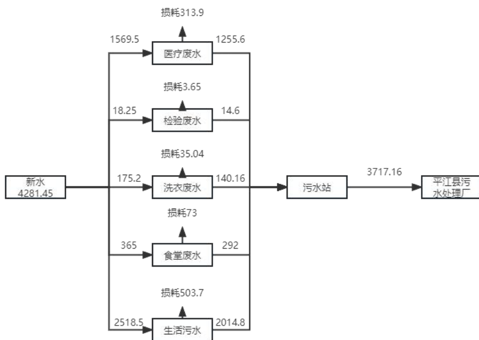
图 2-1 水平衡图 单位 \text{m}^3/\text{a}
