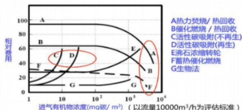
图 6.1-1 常用的有机废气处理工艺适用浓度及运行费用对比图
