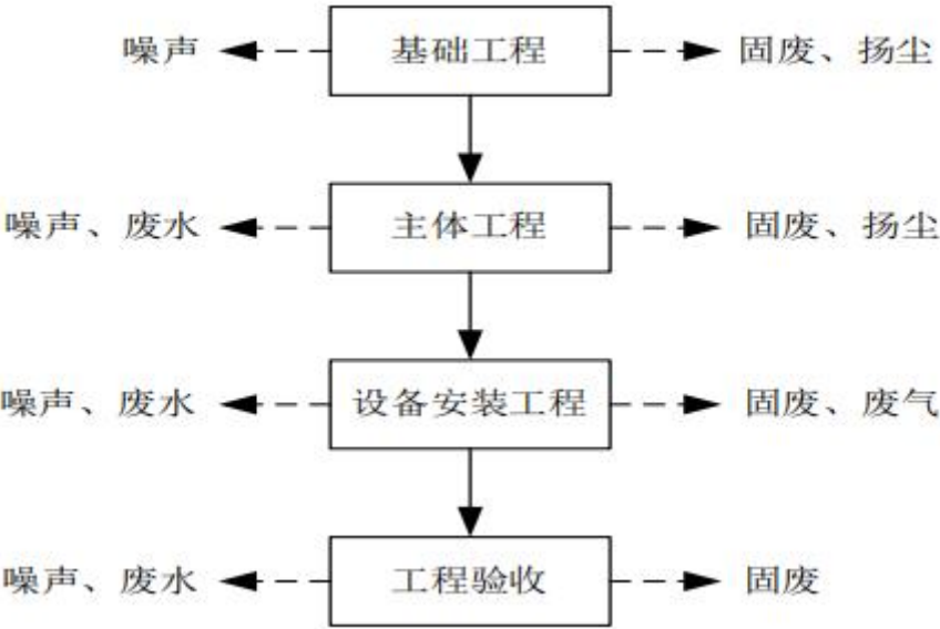
图 5.2-1 施工期工艺流程及产污节点
