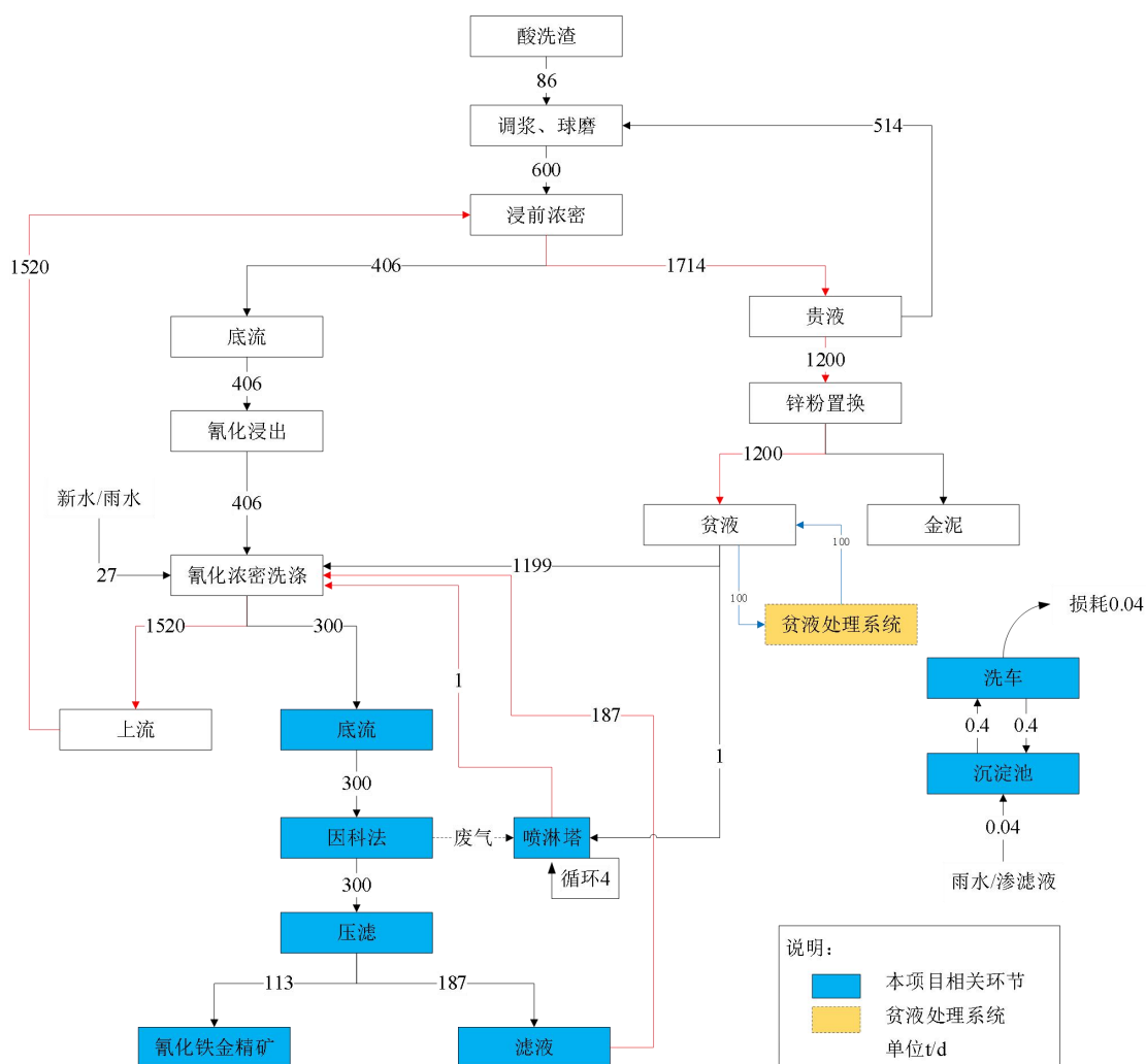
图 1 水平衡图
