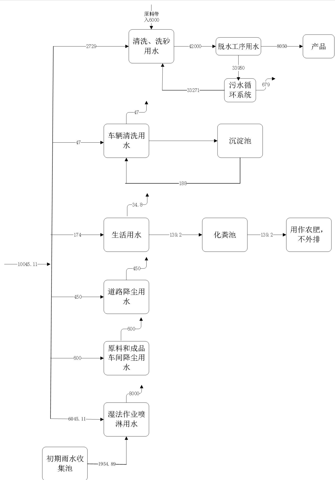
图 2-1 水平衡图 单位 t/a
