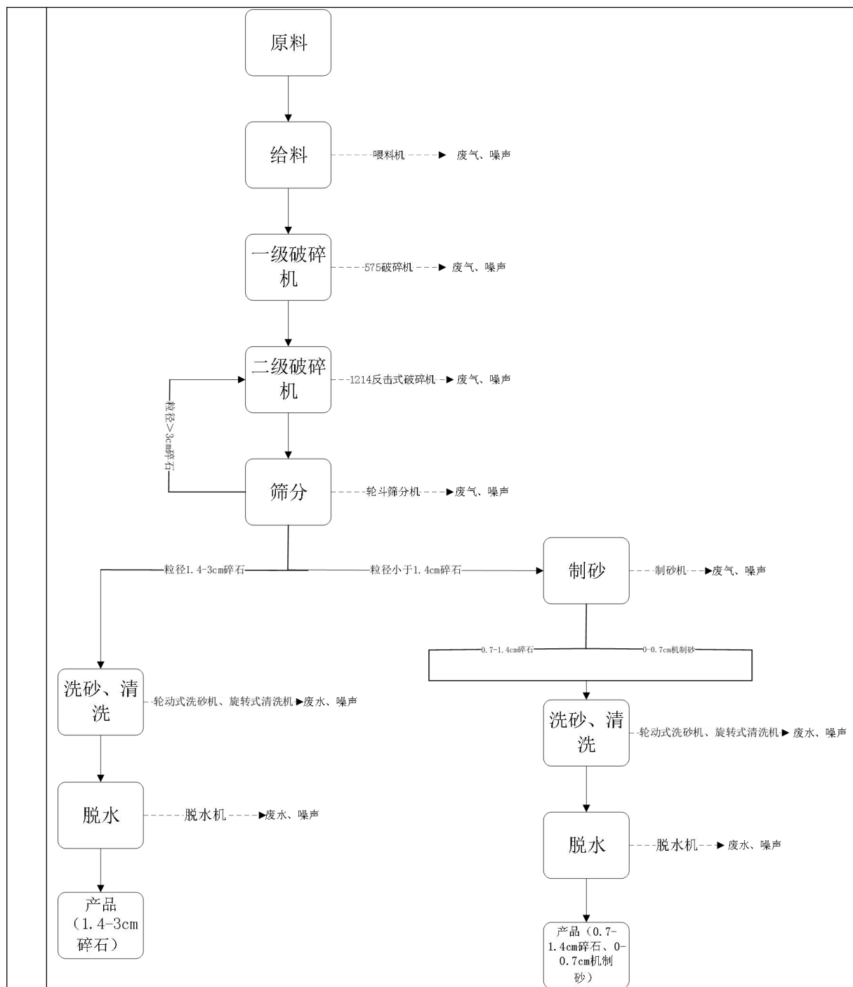
图 2-3 建设项目工艺流程及产污环节示意图
