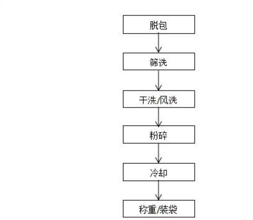
辣椒加工流程图:
