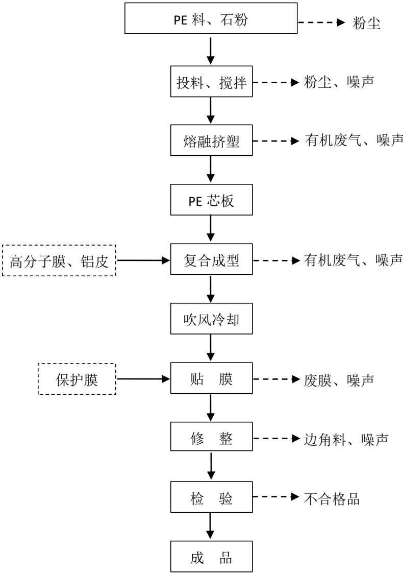
图 2-1 铝塑板生产工艺流程及产污节点图
