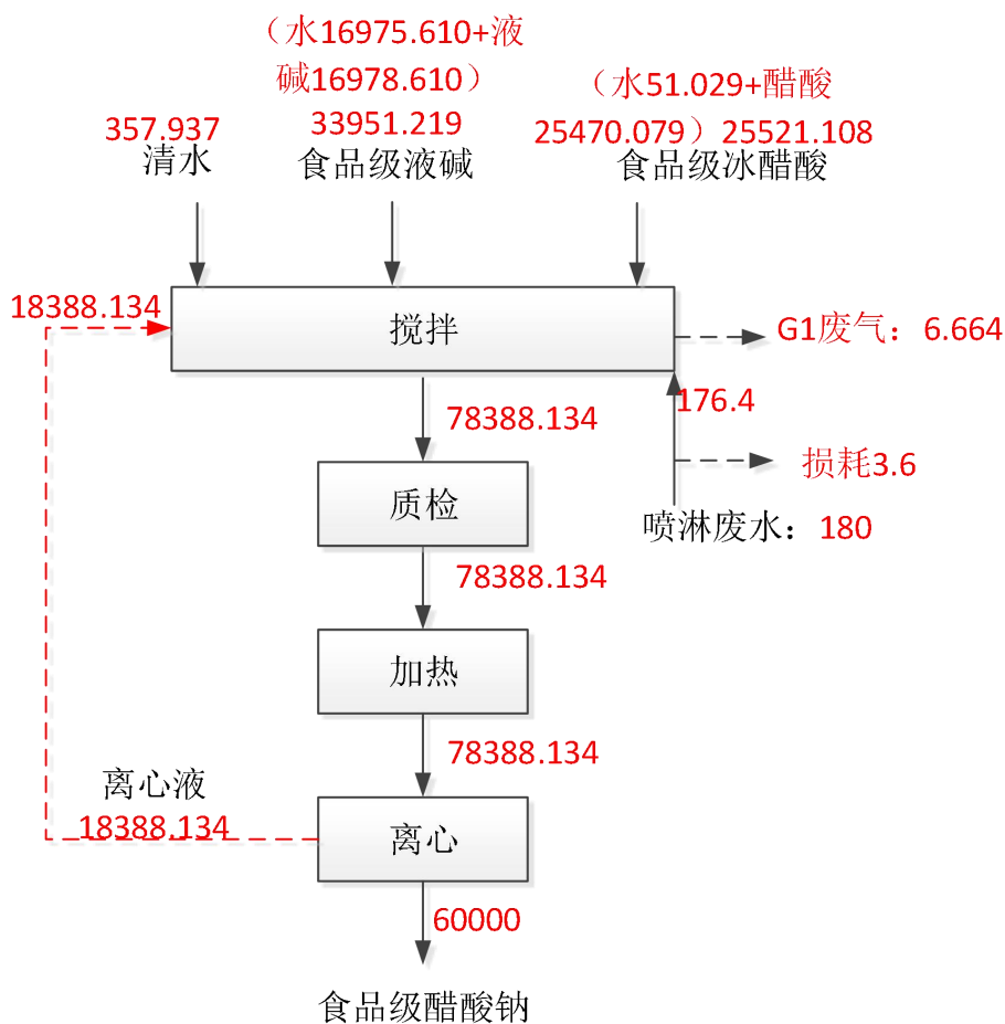
图 2.8-1 物料平衡图
